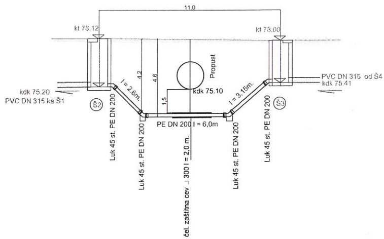
DETALJ SIFONSKOG PROLAZA KANALIZACIJE DN 315 ISPOD PROPUSTA NA MELIORACIONOM KANALU 131 R = 1 : 10
